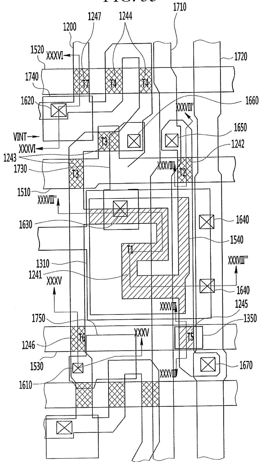
FIG. 33
